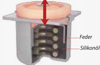
Doppelter Federweg einer herkömmlichen Halterung
